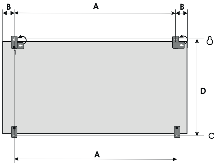
D-FB3 19-xxx Montage mit Hängelaschen
