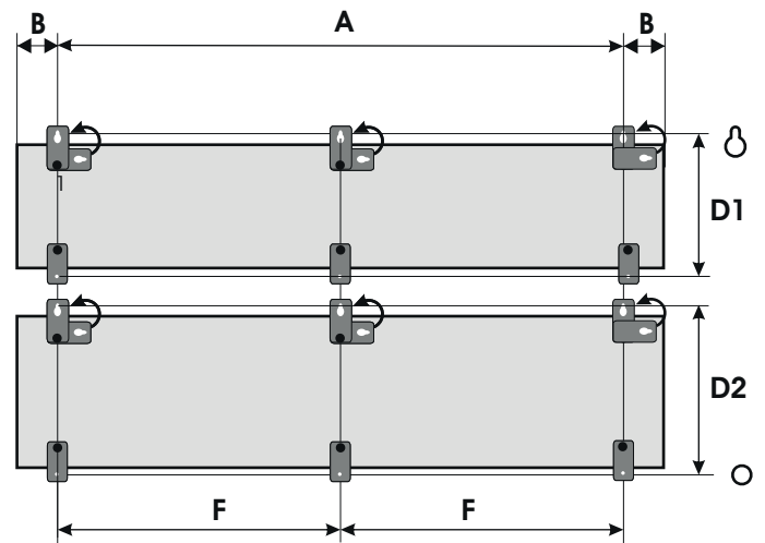
D-FB3 19-xxx Montage mit Hängelaschen
