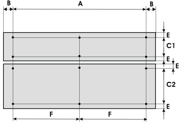
D-FB3 19-xxx Montagelöcher - alle mit M6
