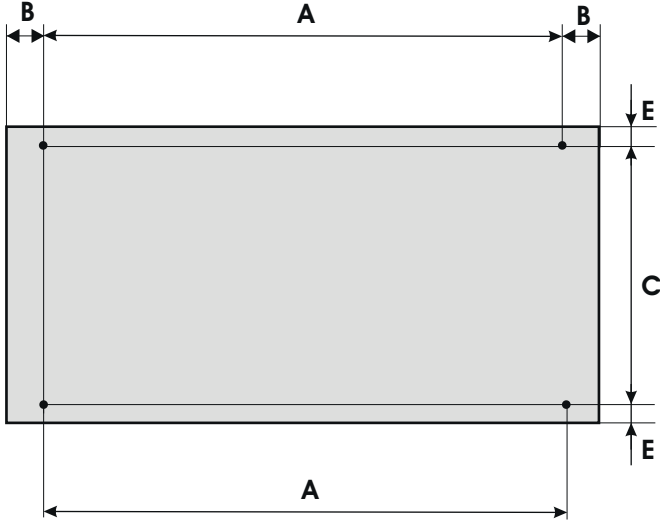
D-FB3 19-xxx Montagelöcher - alle mit M6
